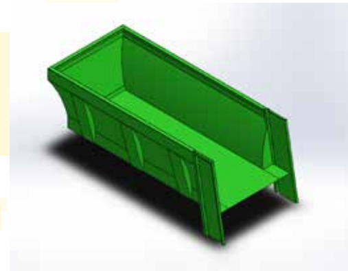
• Plano caja de Tritón 150 Tritón 150 box design
