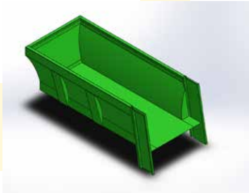
• Plano caja de Tritón 120 Tritón 120 box design
