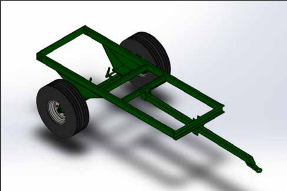
1 Eje de tubo estructural 1 essieu châssis en tube structurel
